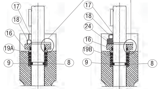
Zebra-CL™: Type 0A, 1A
